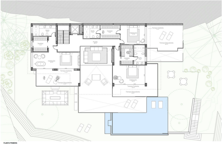
PLANTA PRIMERA 1:100
