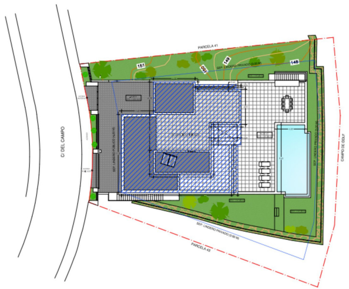
ORDENACIÓN GENERAL DE PARCELA: EMPLAZAMIENTO ACOTADO
