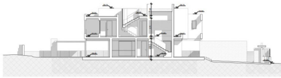
SECCIÓN A-A'
